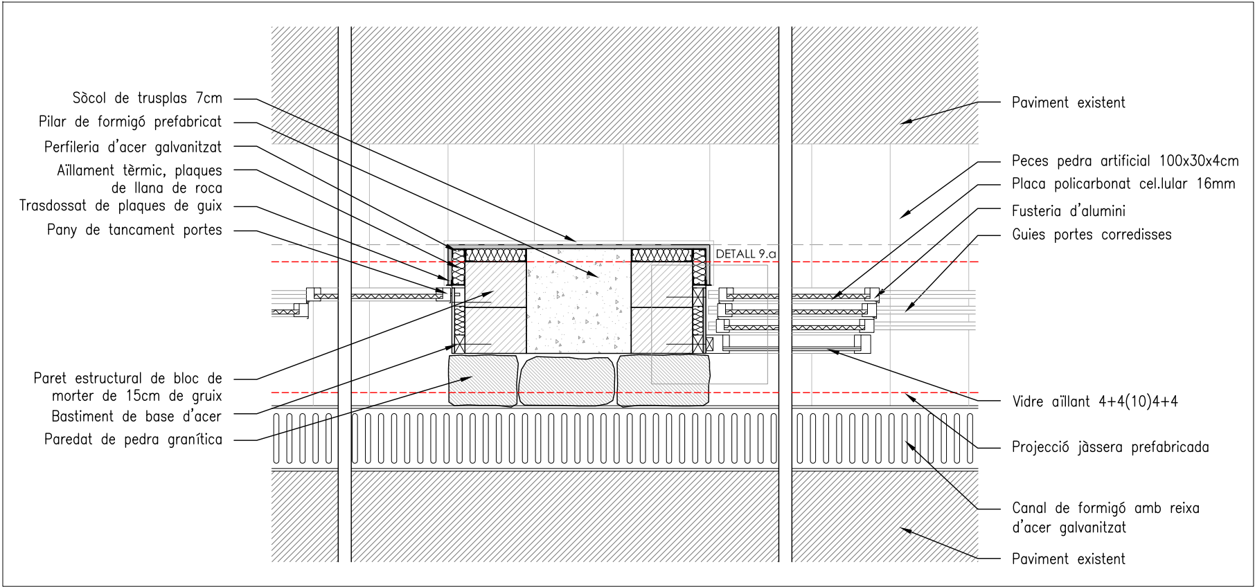
DETALL 5 (Pilar Planta Baixa)
