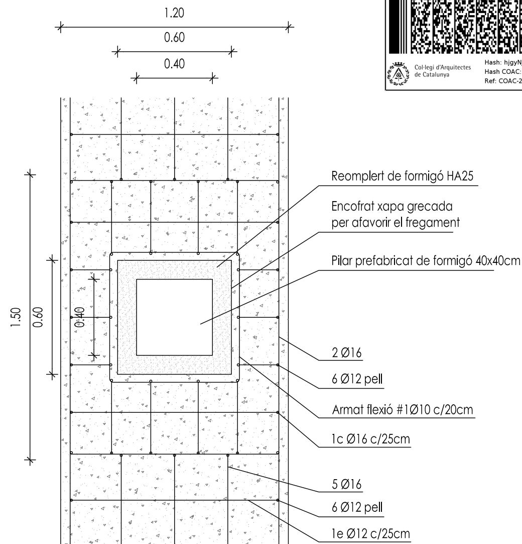
SECCIÓ SABATA CORREGUDA (ZONA PILARS)
