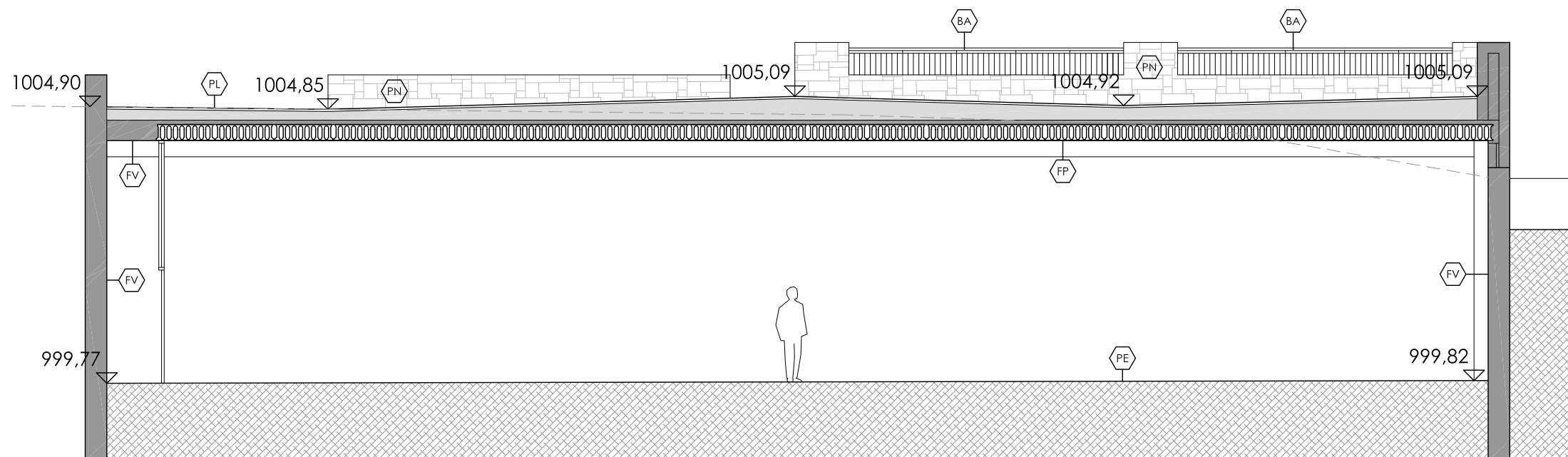
SECCIÓ LONGITUDINAL
