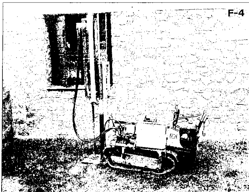
Fotografies 3 i 4: Zona on es van fer els penetròmetres.
