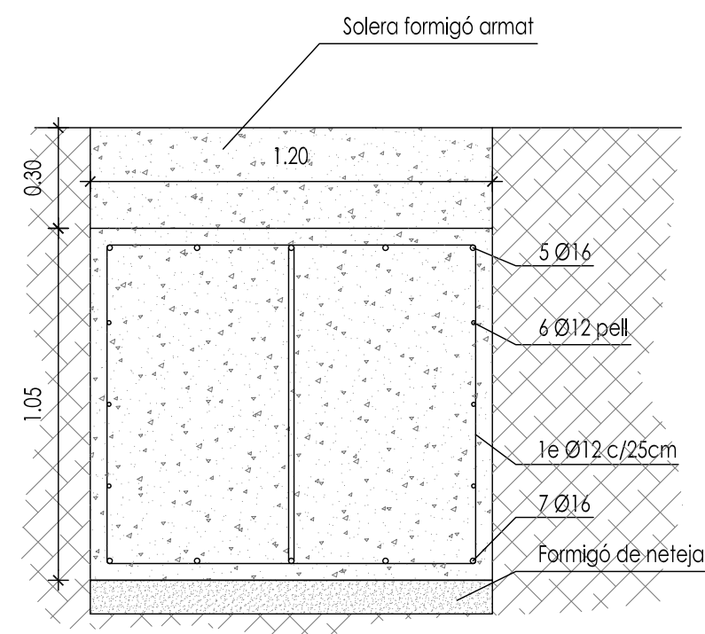
SECCIÓ SABATA CORREGUDA (ZONA ENTRE PILARS)
