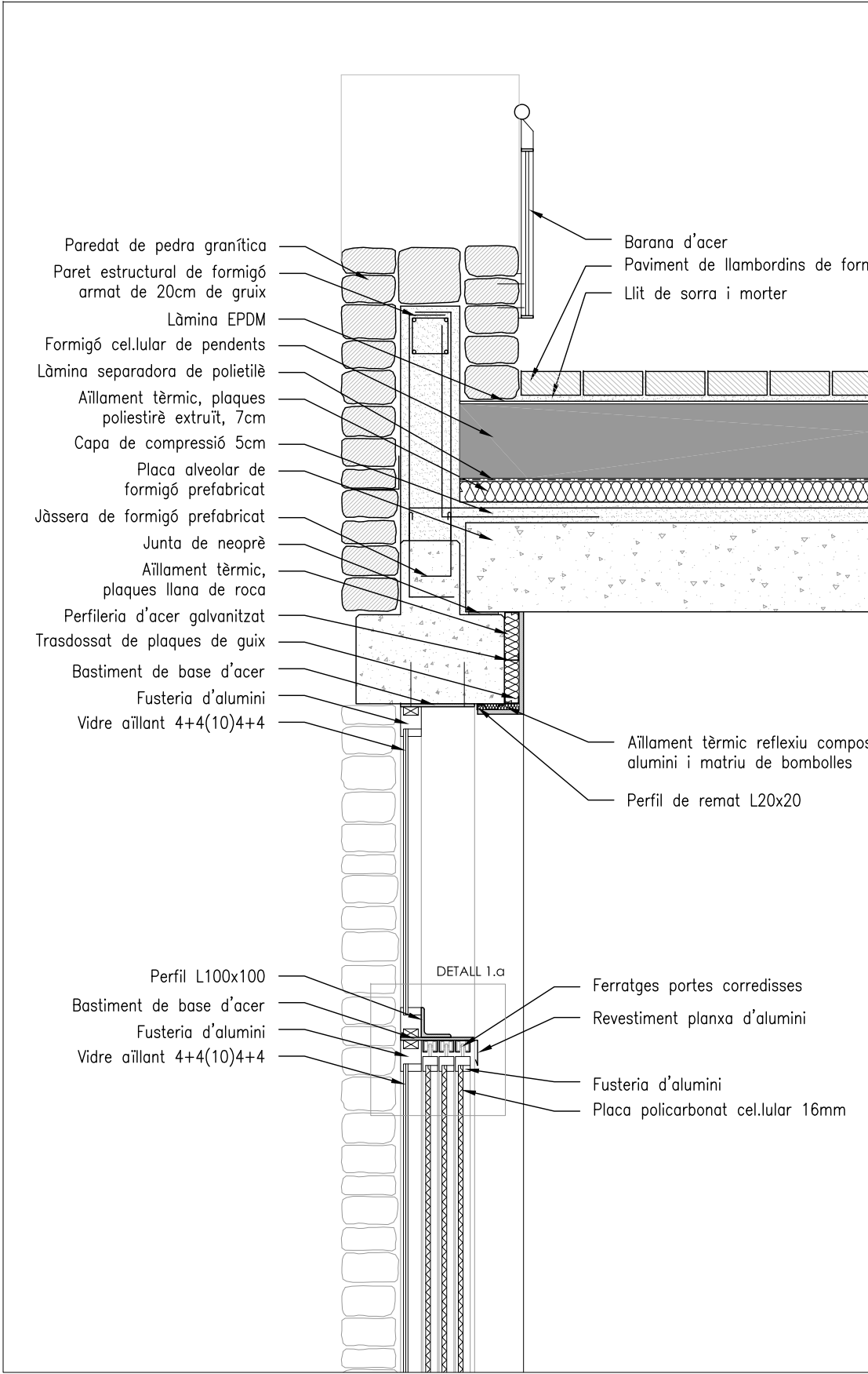
DETALL 1
