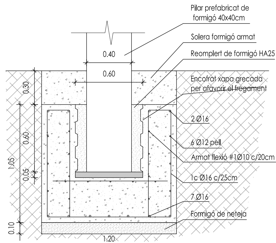
SECCIÓ SABATA CORREGUDA (ZONA PILARS)
