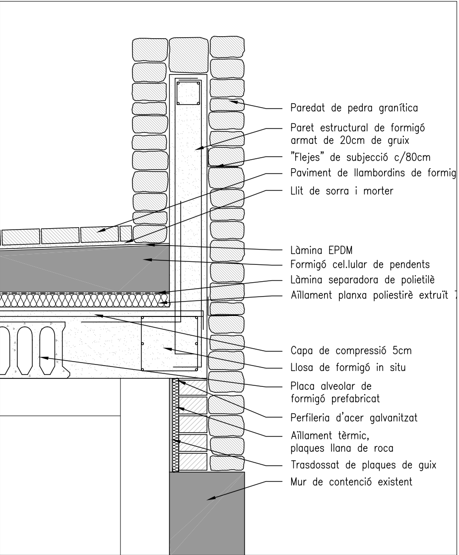
DETALL 3
