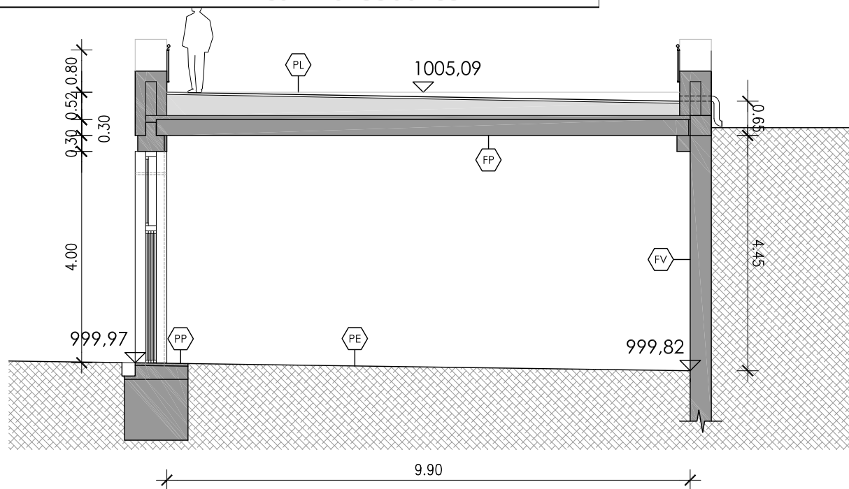
SECCIÓ TRANSVERSAL DESGUÀS PLAÇA
