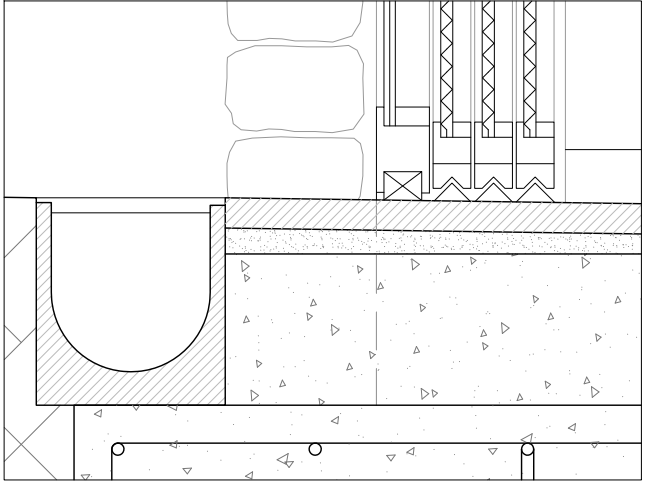
DETALL 2.a
