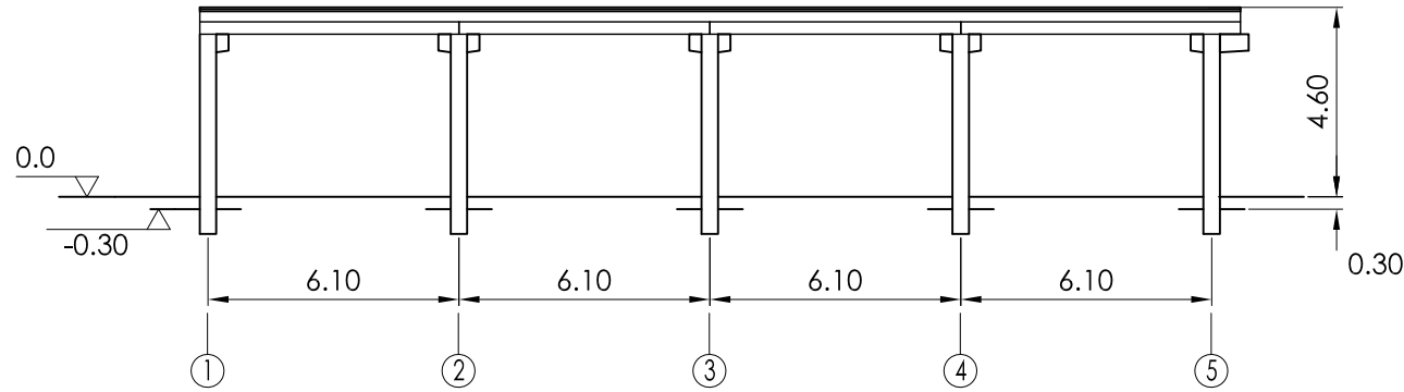
ALINEACION A
