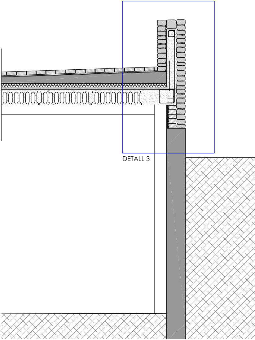
SECCIÓ TRANSVERSAL
