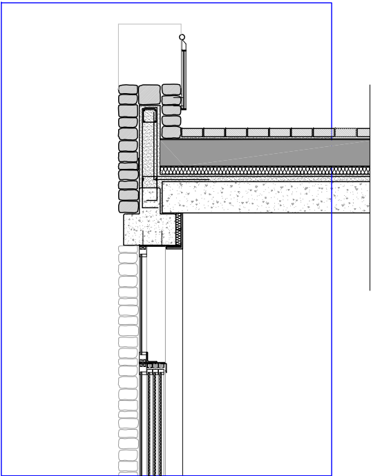
DETALL 1
