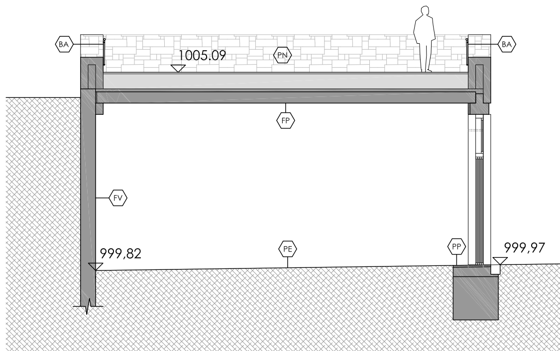
SECCIÓ TRANSVERSAL ALÇAT MUR CARRER
