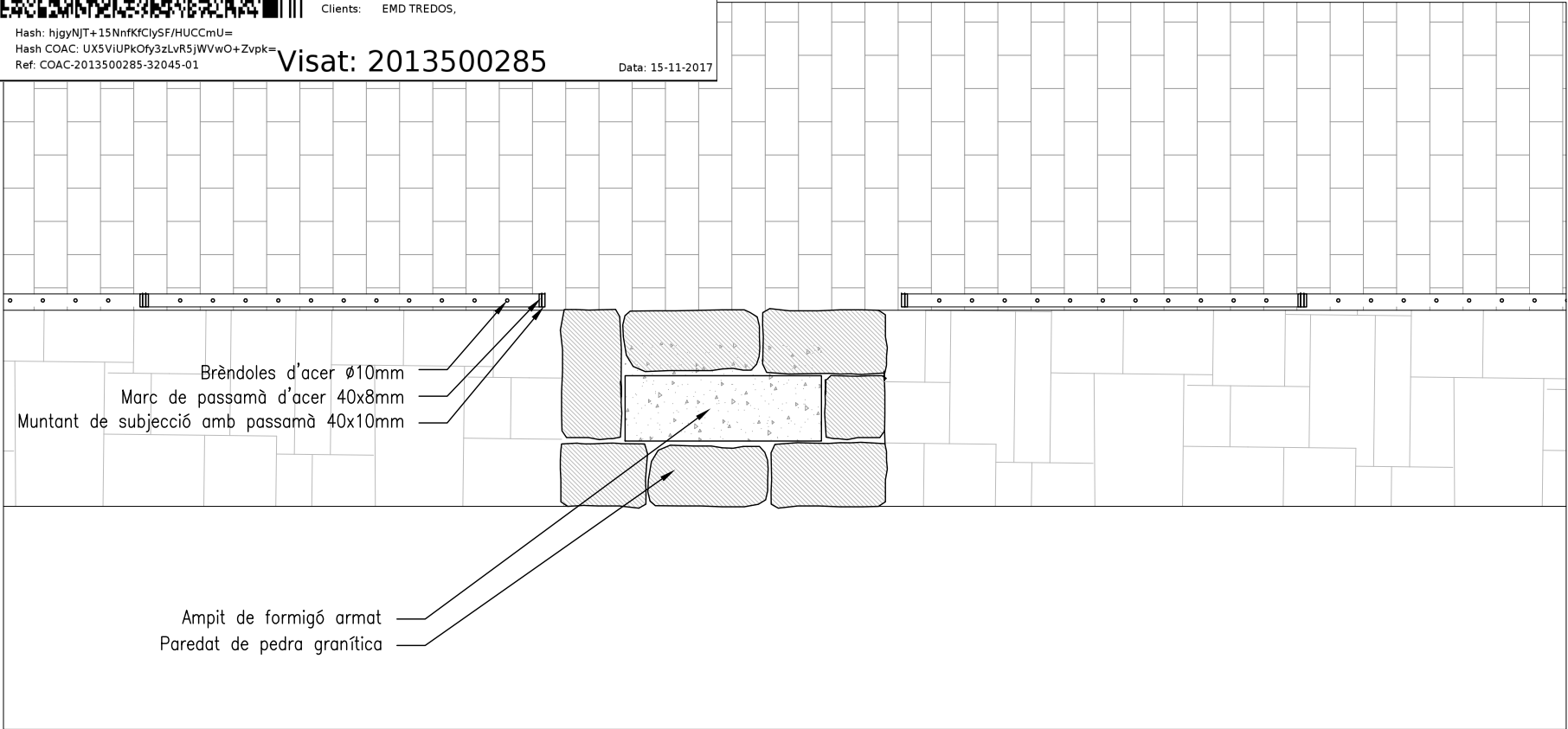
DETALL 4 (Barana Planta Primera)
