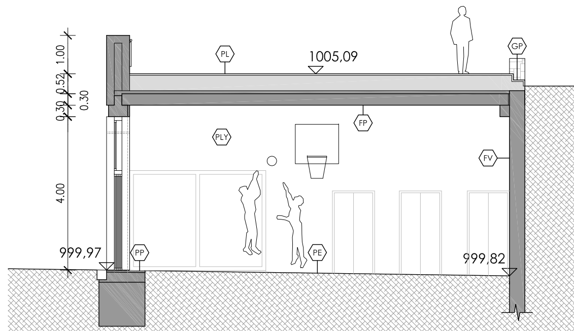
SECCIÓ TRANSVERSAL ACCÉS PLAÇA ESCALA
