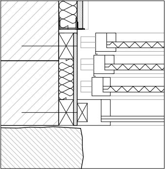
DETALL 5.a
