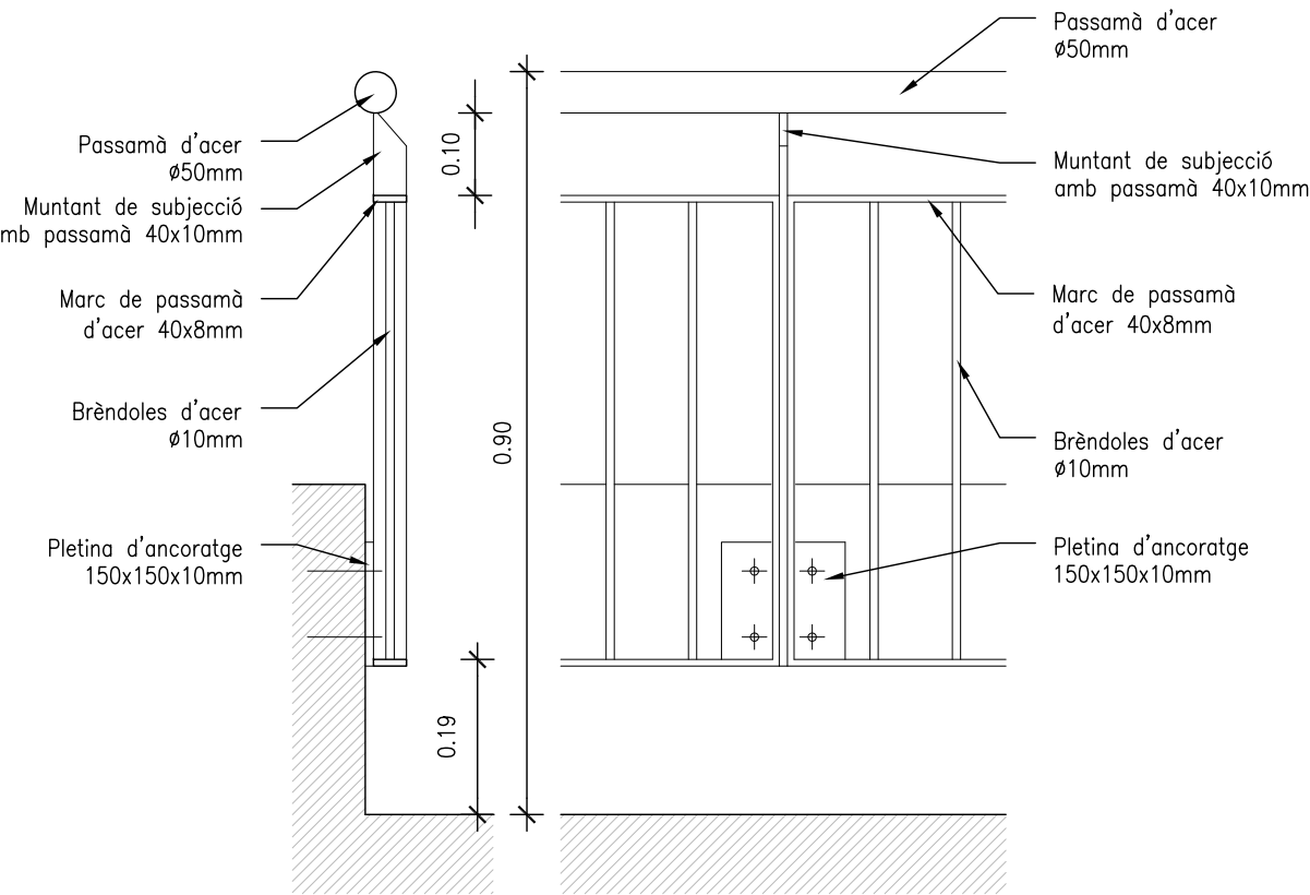
Barana plaça exterior
