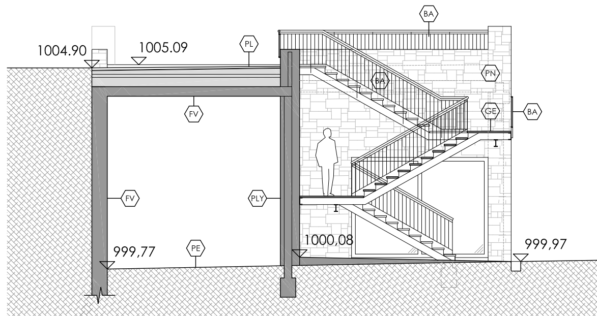
ALCAT ESCALA EXTERIOR
