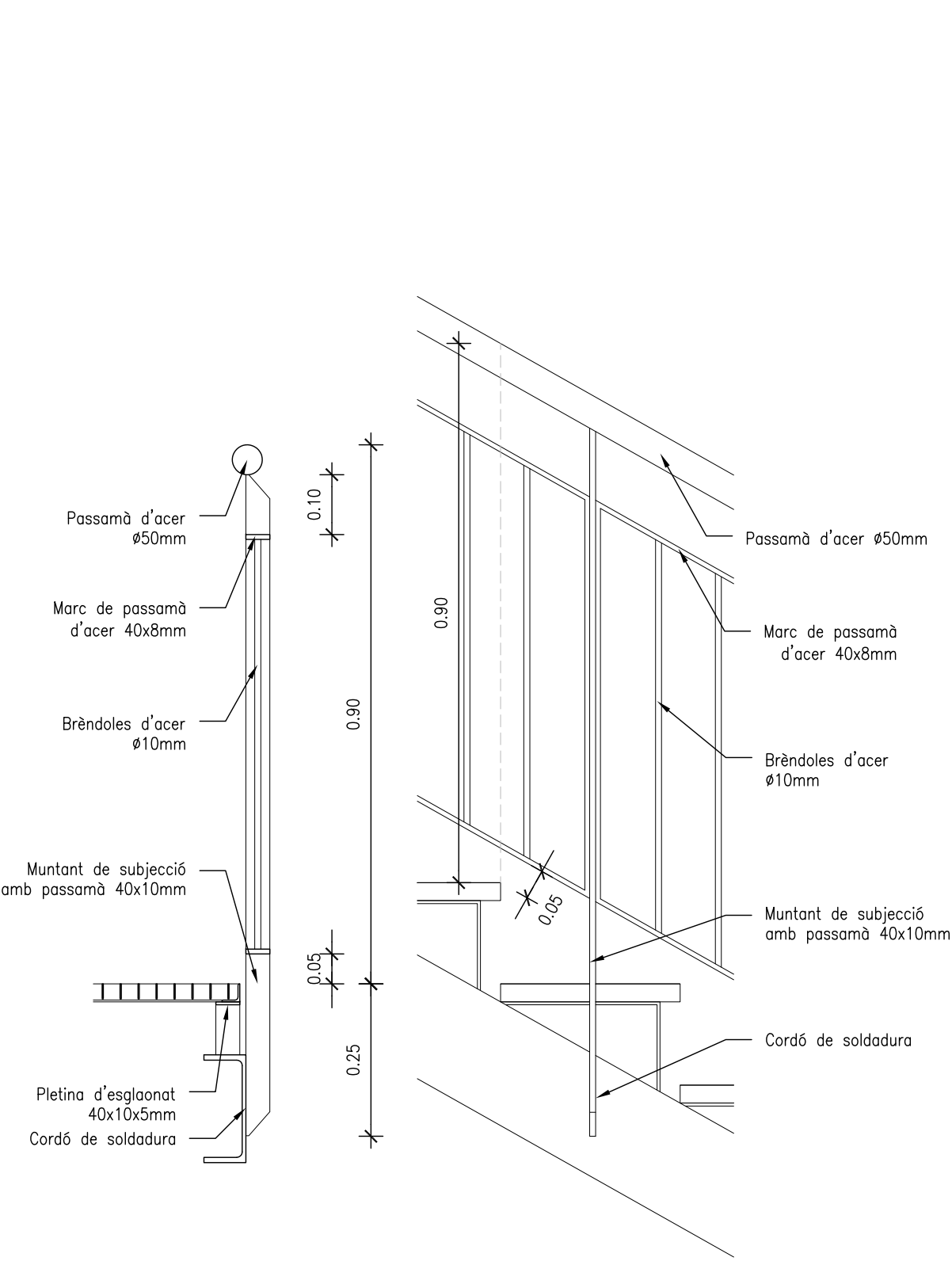
Barana escala exterior
