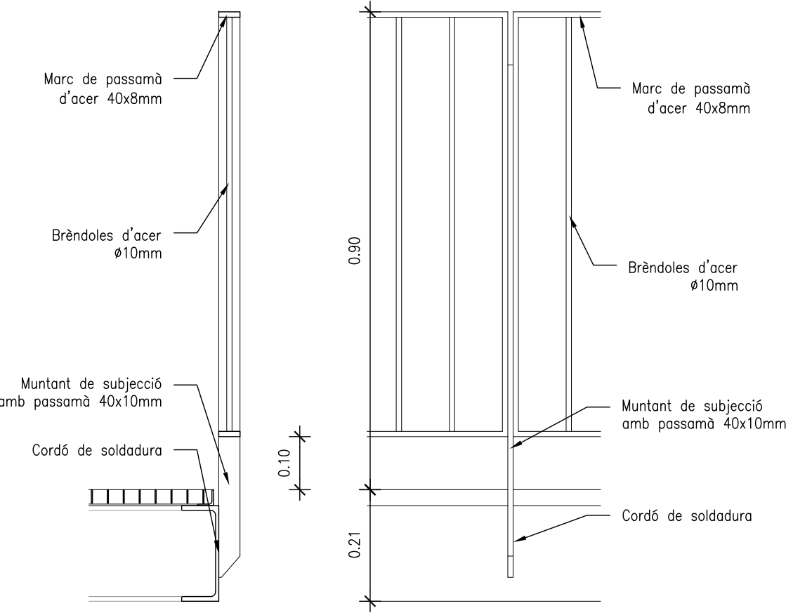
Barana replà escala exterior
