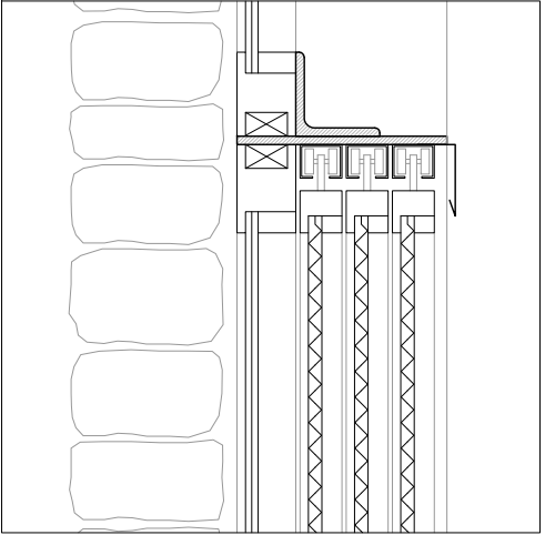
DETALL 1.a
