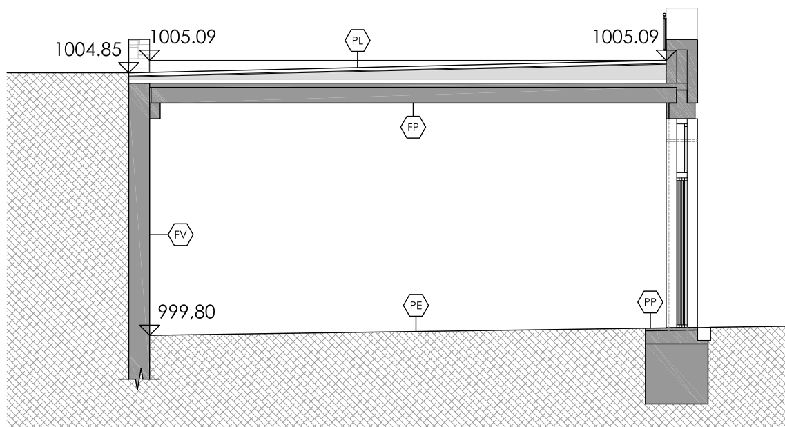
SECCIÓ TRANSVERSAL ACCÉS PEATONAL PLAÇA
