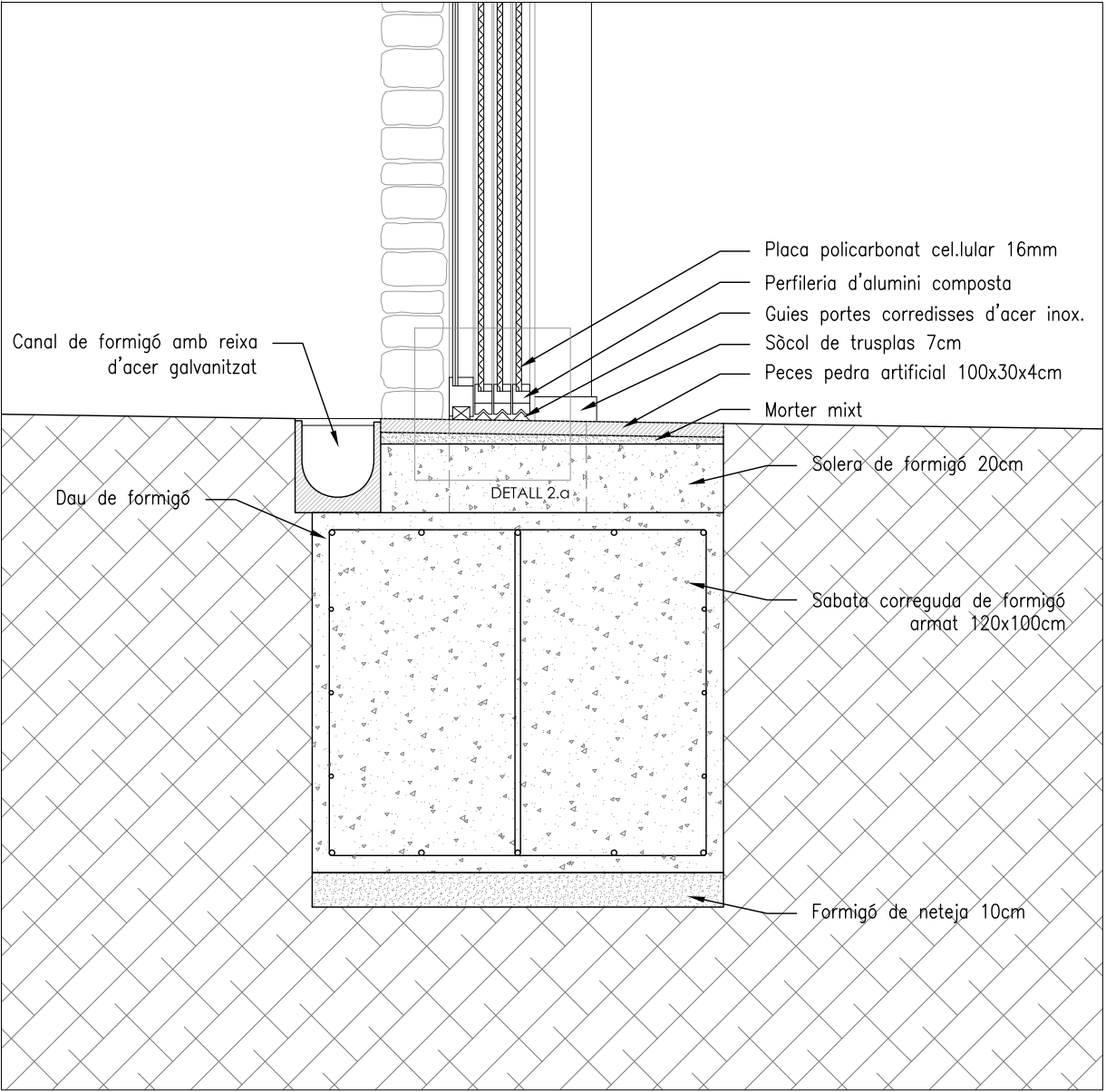
DETALL 2
