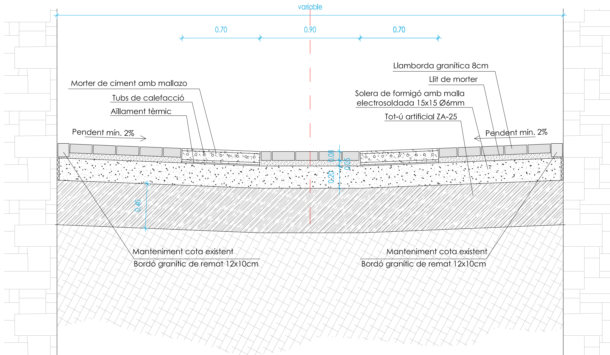
SECCIÓ TIPUS ZONA RODERES
