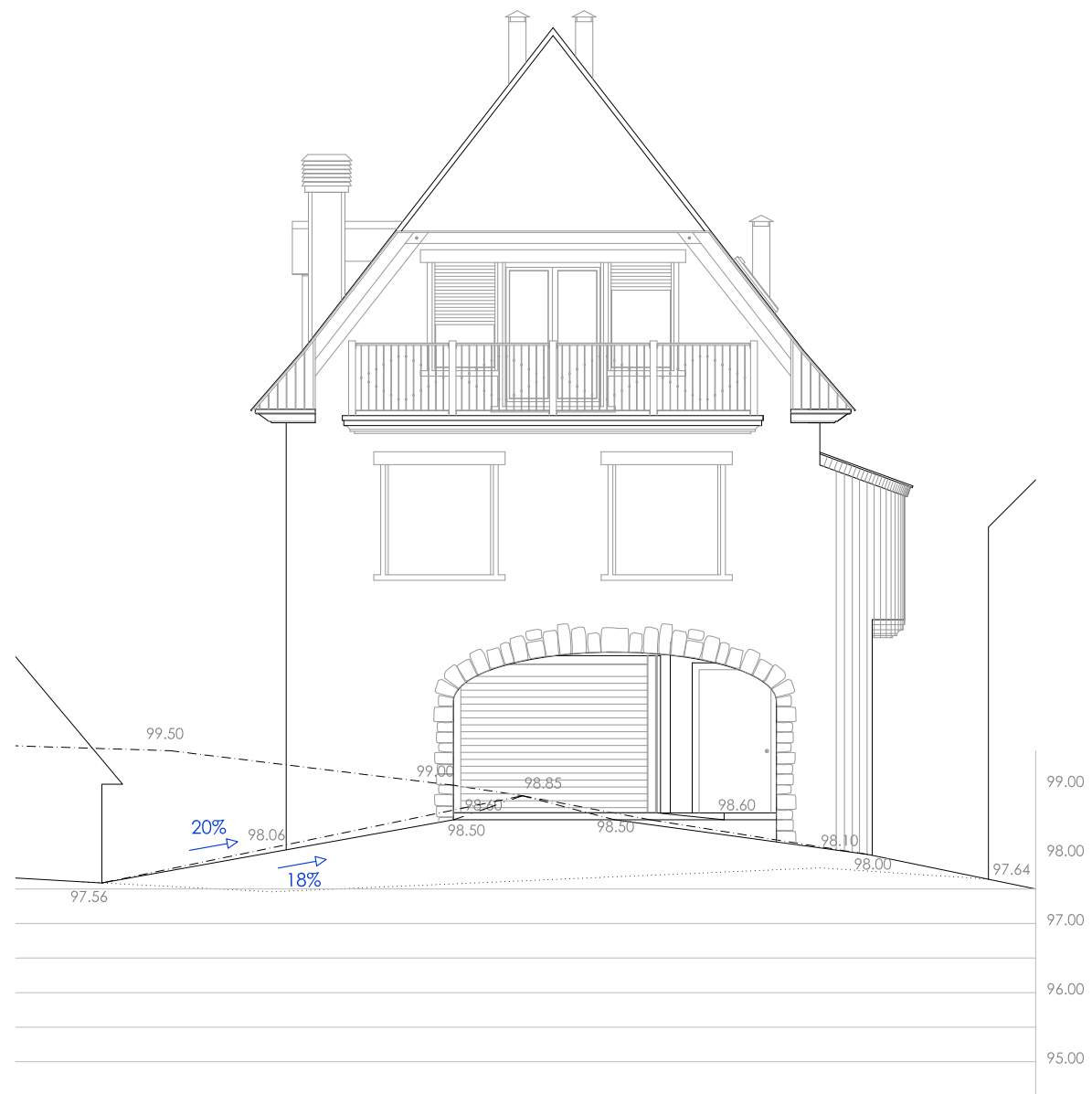
ALÇAT CARRER SANT ANDREU
