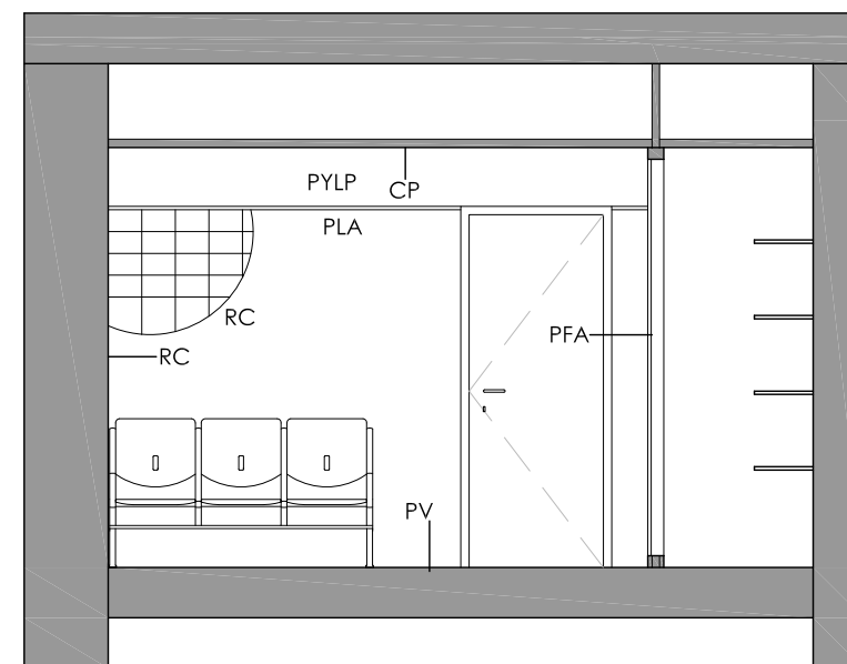
Secció 5
