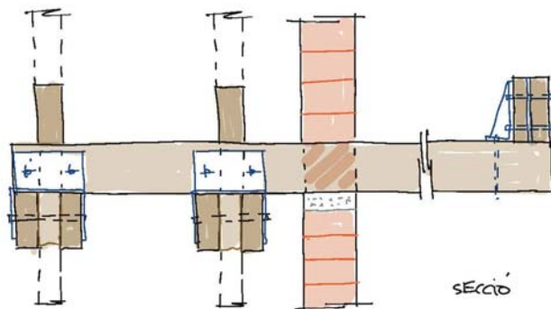
DETALL 4
