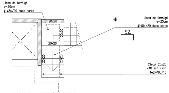
ESCALA SP1 E: 1/50
