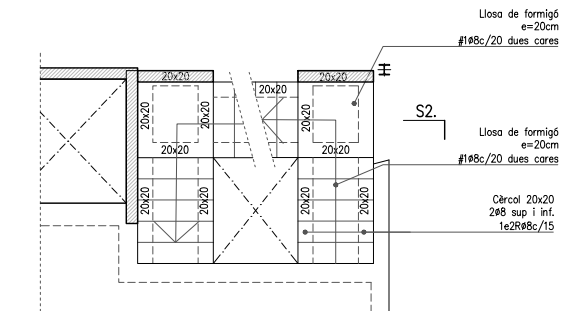
ESCALA SPB E: 1/50
