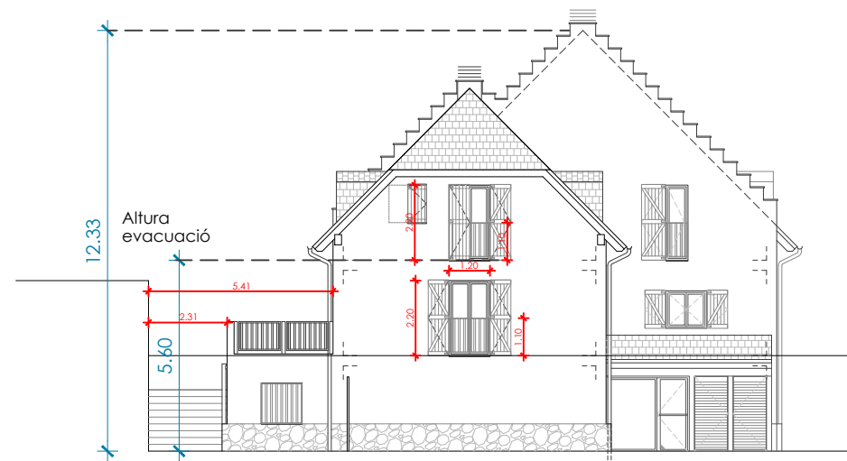
Alçat tester
