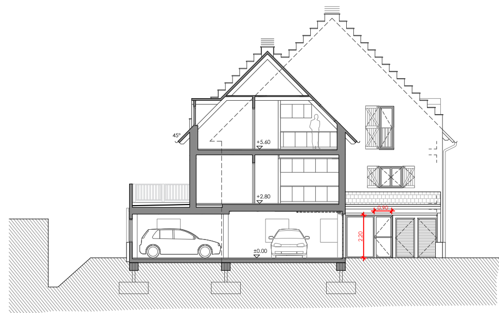
Alçat principal
