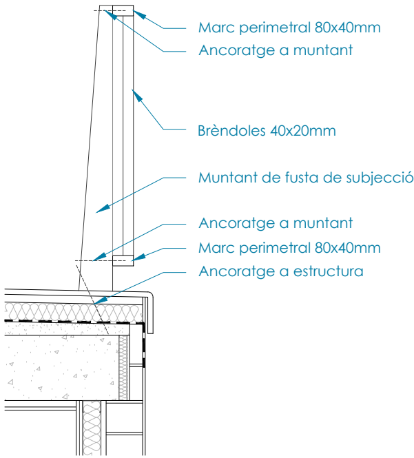
BARANES DE FUSTA EXTERIORS
