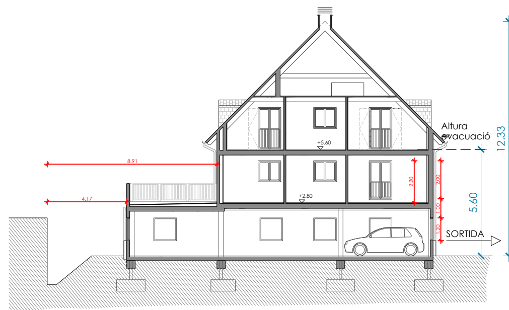
Secció transversal
