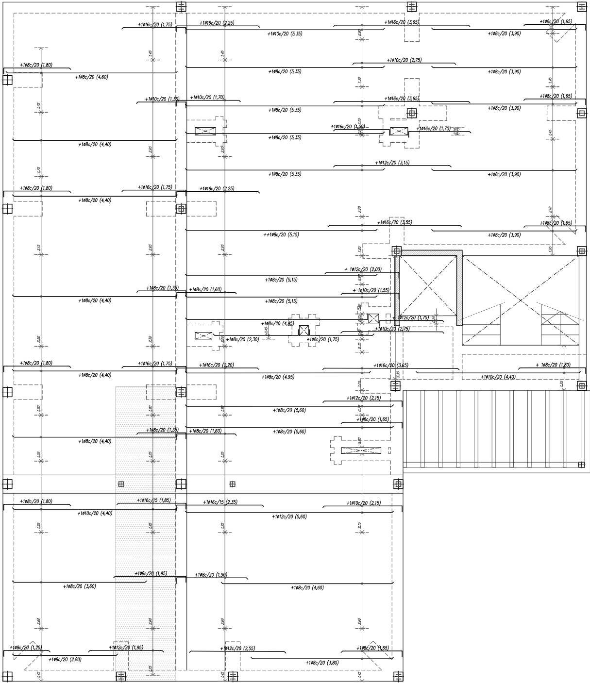
SOSTRE PLANTA BAIXA E: 1/50
