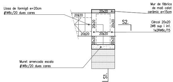
ARRENCADA ESCALA E: 1/50
