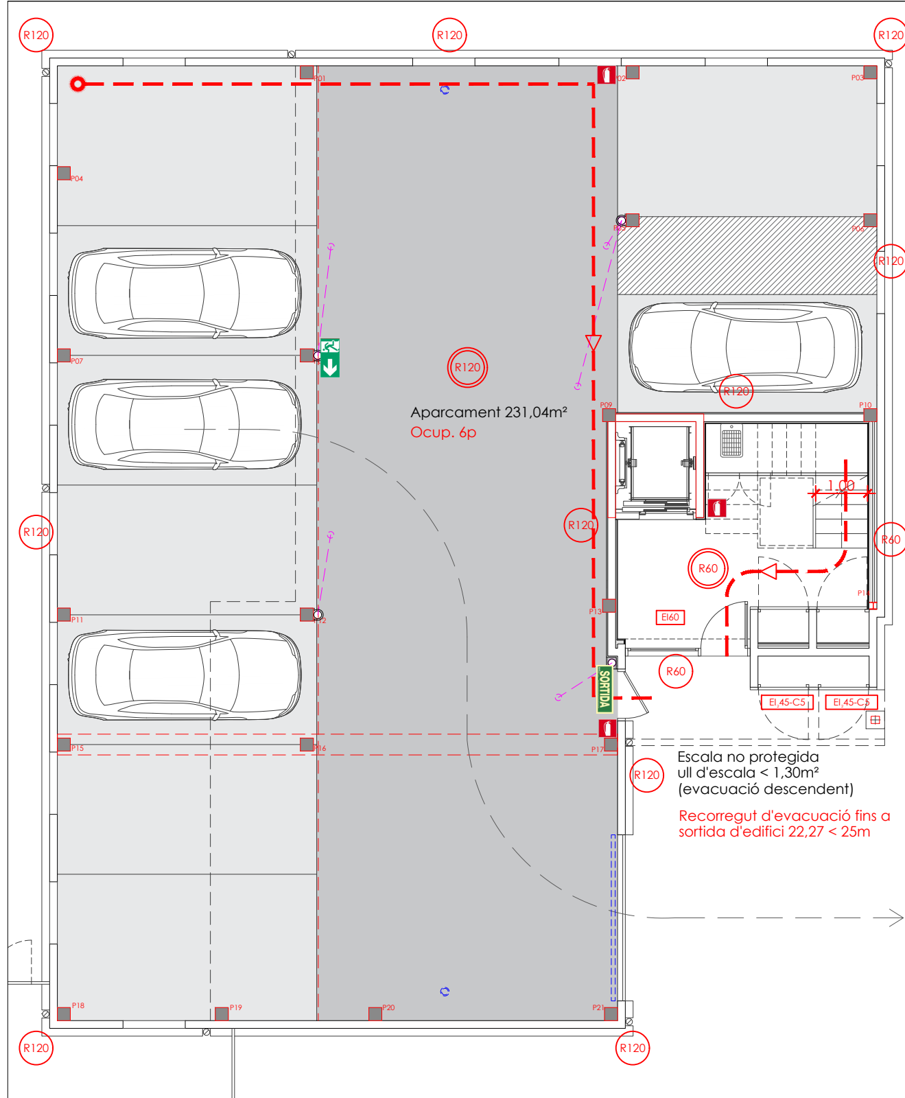
Planta Baixa
