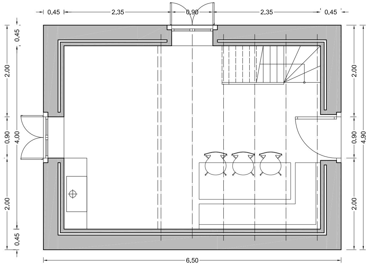
PLANTA BAIXA
