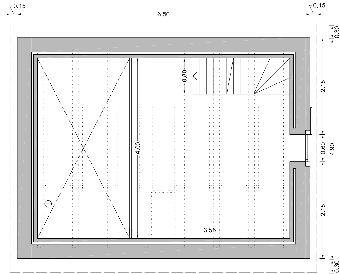
PLANTA HUMARAU
