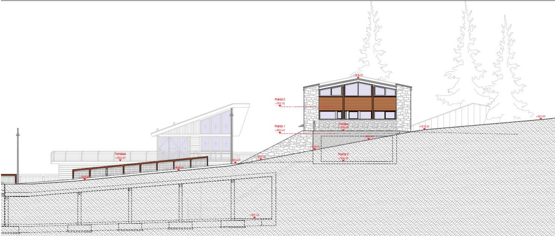
ESTAT ACTUAL
