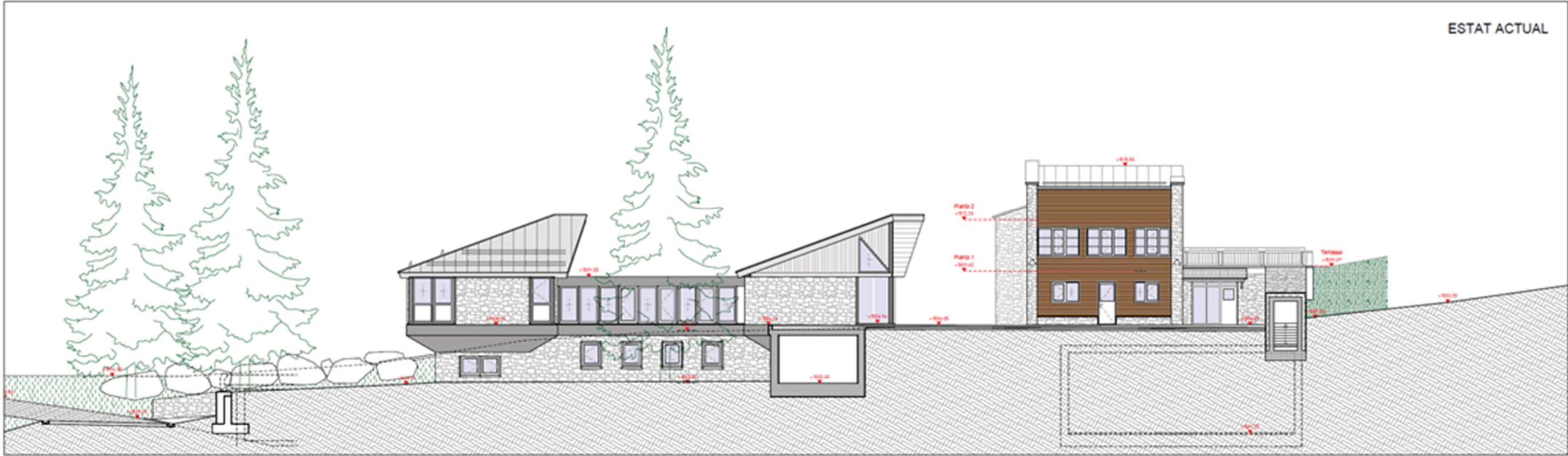
ALÇAT SUD
