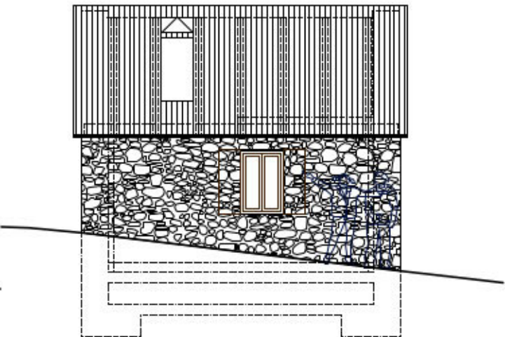
FAÇANA SO
