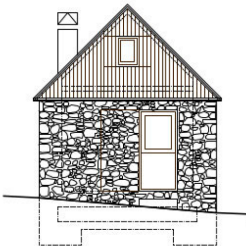
FAÇANA SE
