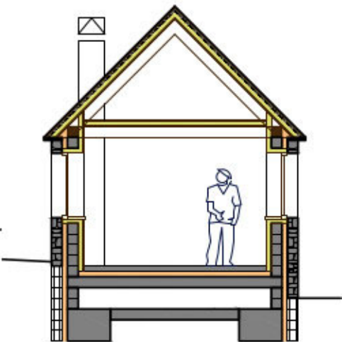
SECCIO TRANSVERSAL
