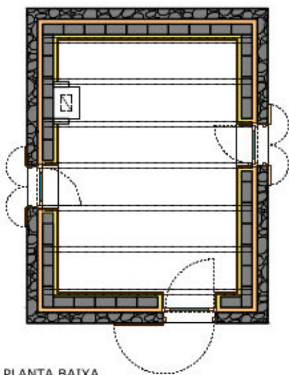
PLANTA BAIXA
