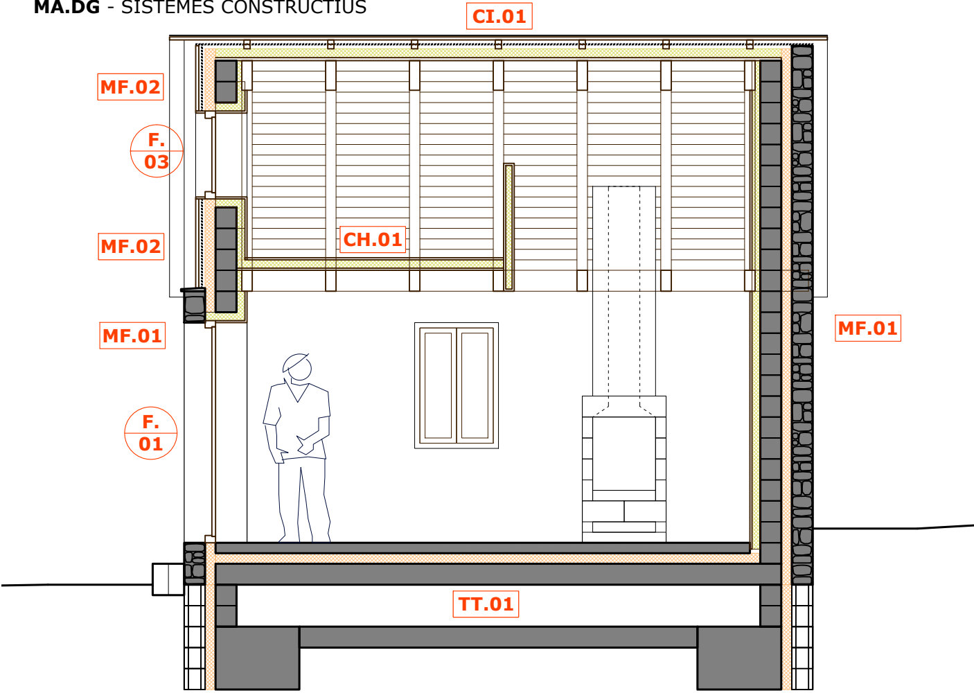
SECCIÓ LONGITUDINAL
