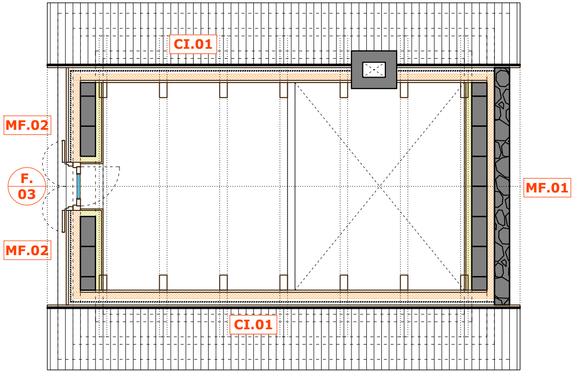
PLANTA ALTELL
