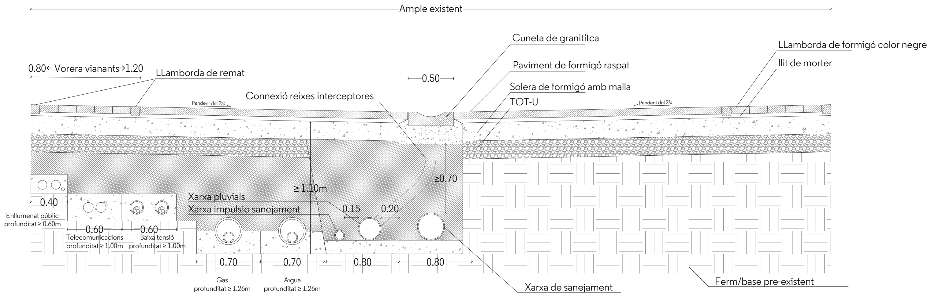
SECCIÓ FERM S1
